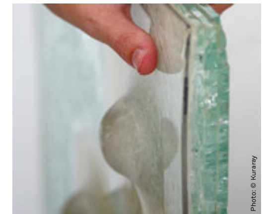
• Trosifol® Spallshield® CPET impact test
